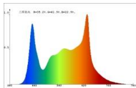
光波長図
