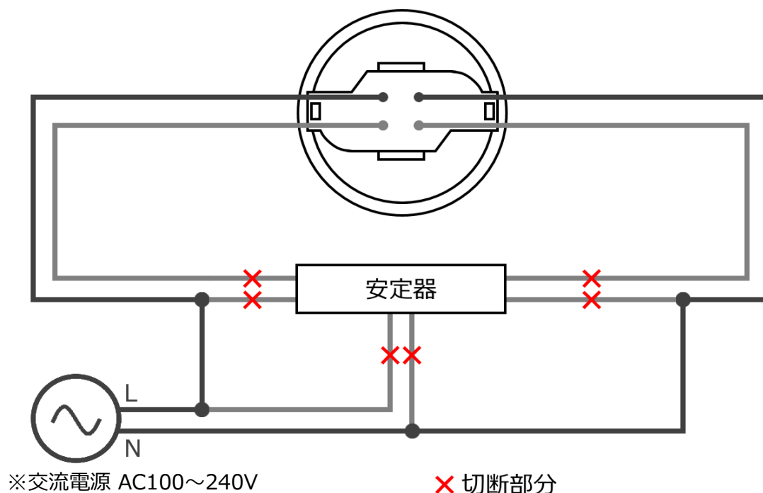
コンパクト型LEDランプFDL型
