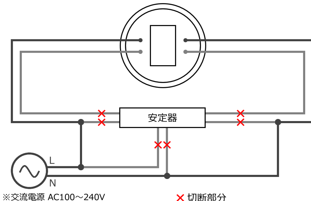
コンパクト型LEDランプFHT型
